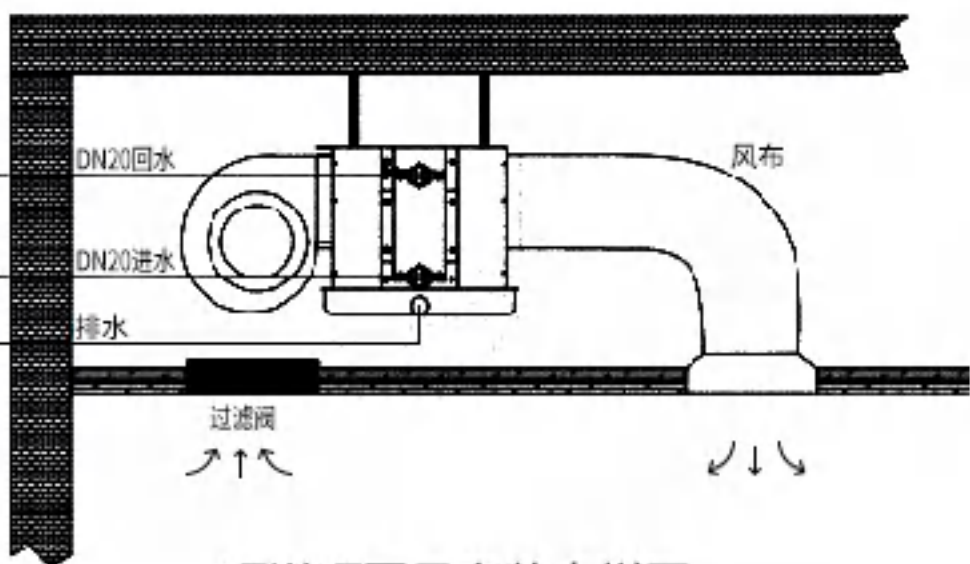
顶送顶回风安装大样图
