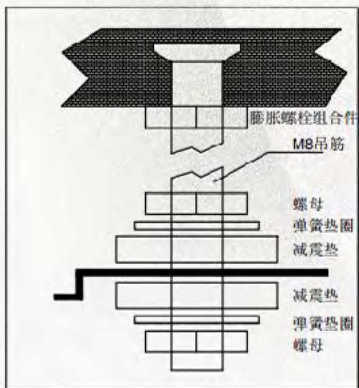
风盘吊装架大样图
