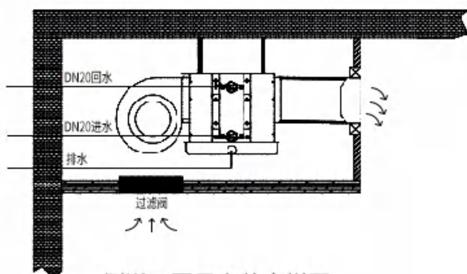
侧送下回风安装大样图
