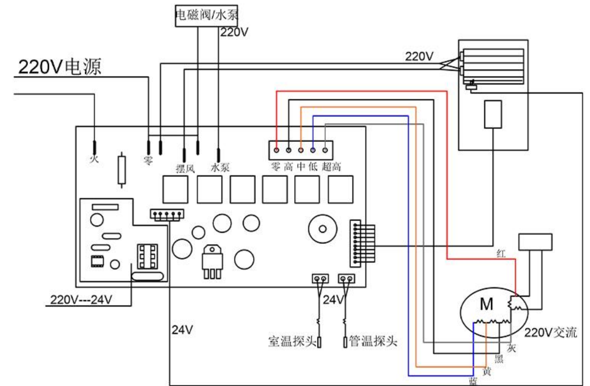
柜机接线原理图
