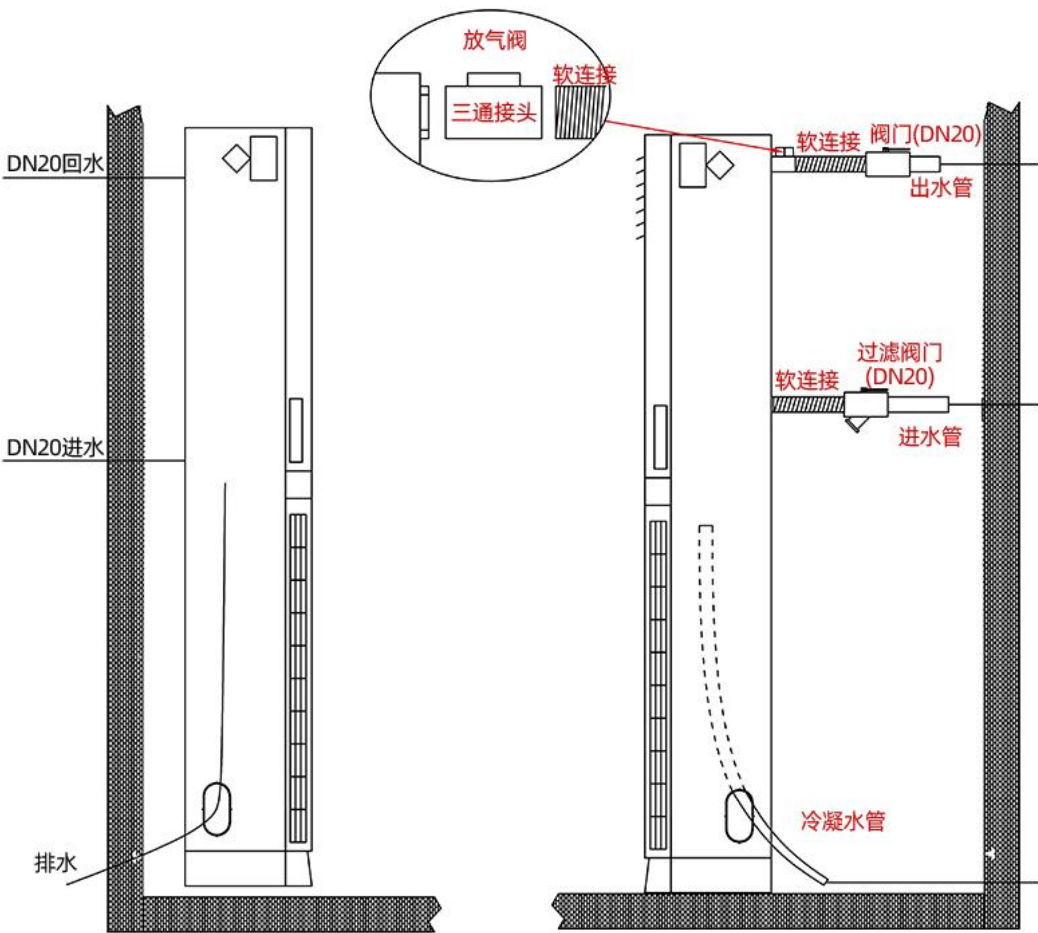
柜机放置大样图
