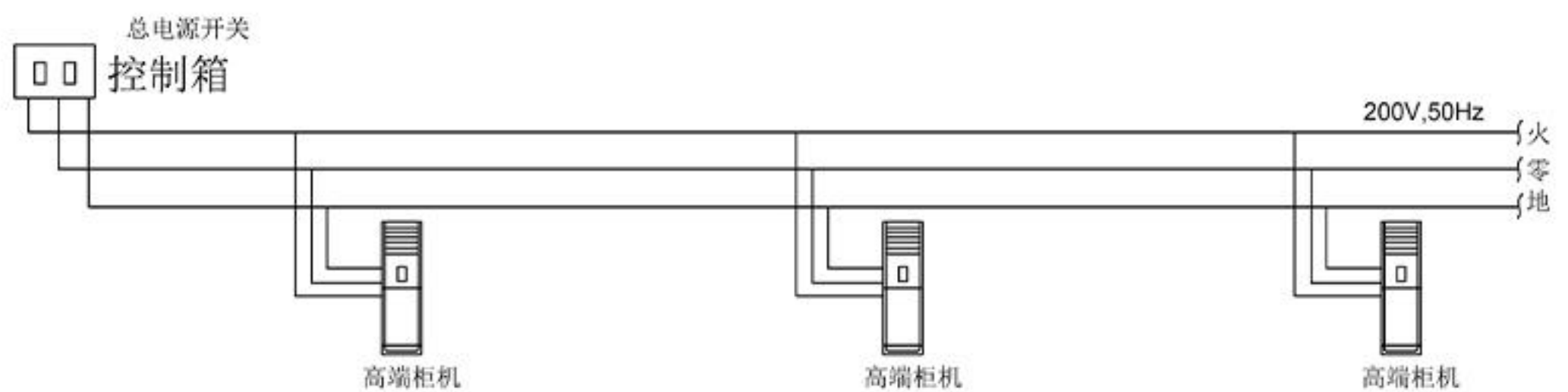
柜机用电源远端接线原理图
